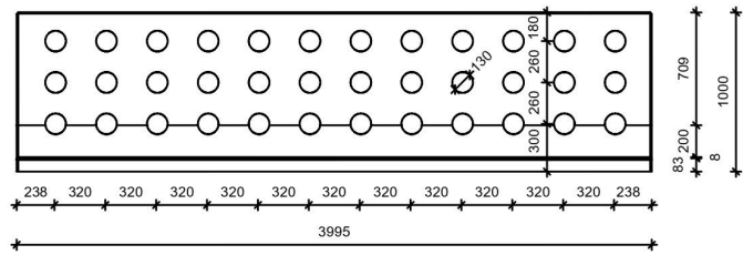
Bovenaanzicht
