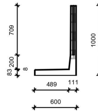
Zij aanzicht
