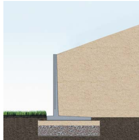
► GRONDKERING MET TALUD
