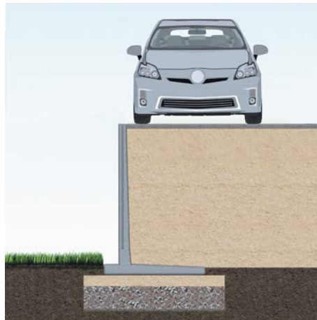
► LICHT VERKEERSBELASTING - A
