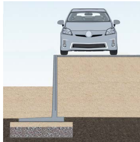
► LICHT VERKEERSBELASTING - B
