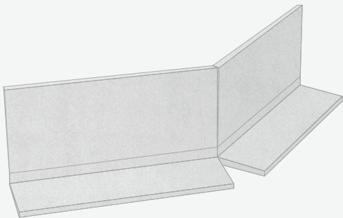
HOEKOPLOSSING IN VERSTEK UITWENDIG
