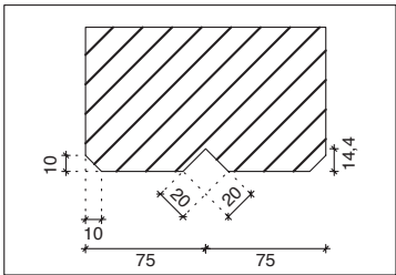
Detail van de uitsparing van de koppelstang
