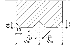
Koppelbuis-sparing
