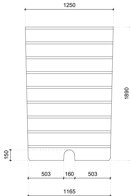
Vooraanzicht
