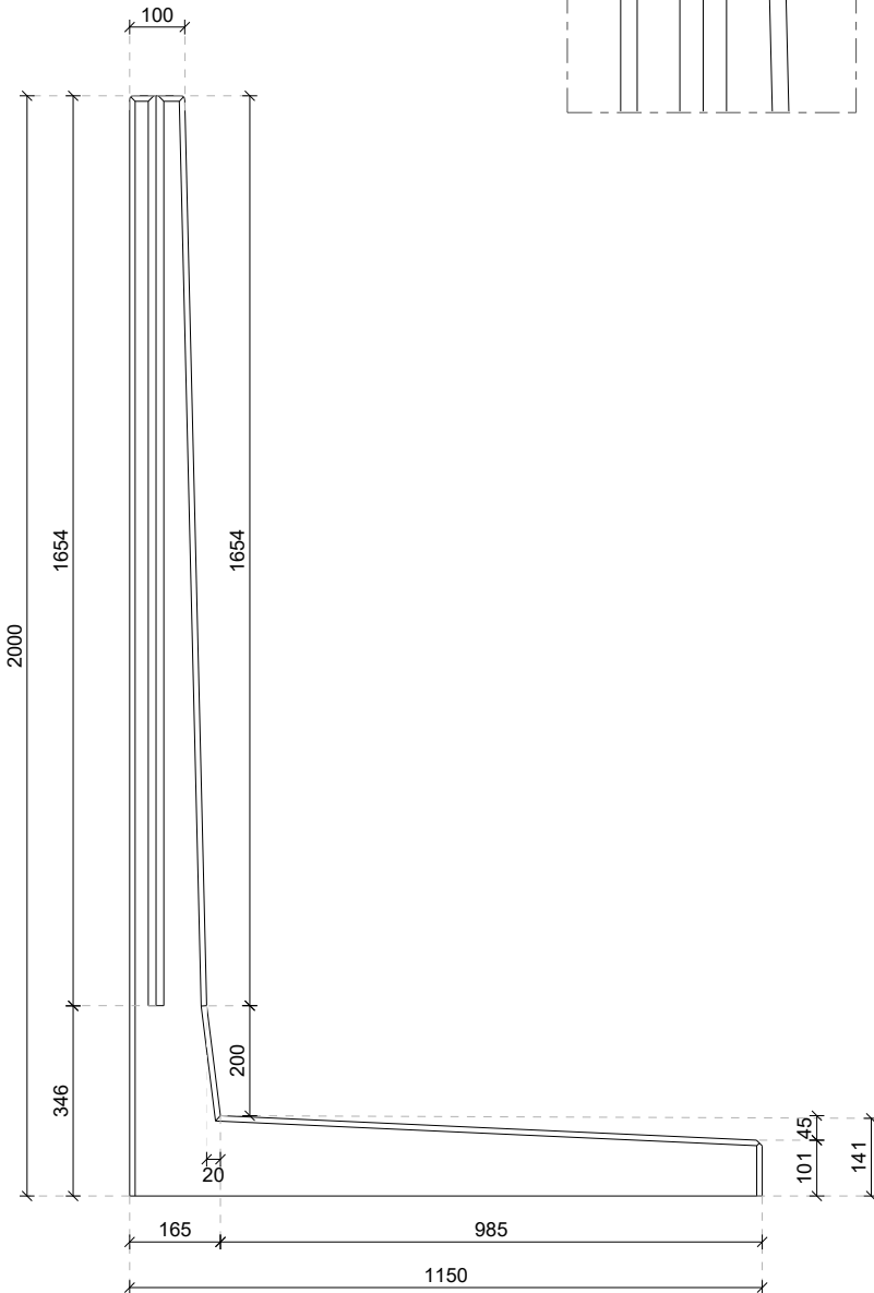
Afgeronde bovenzijde
