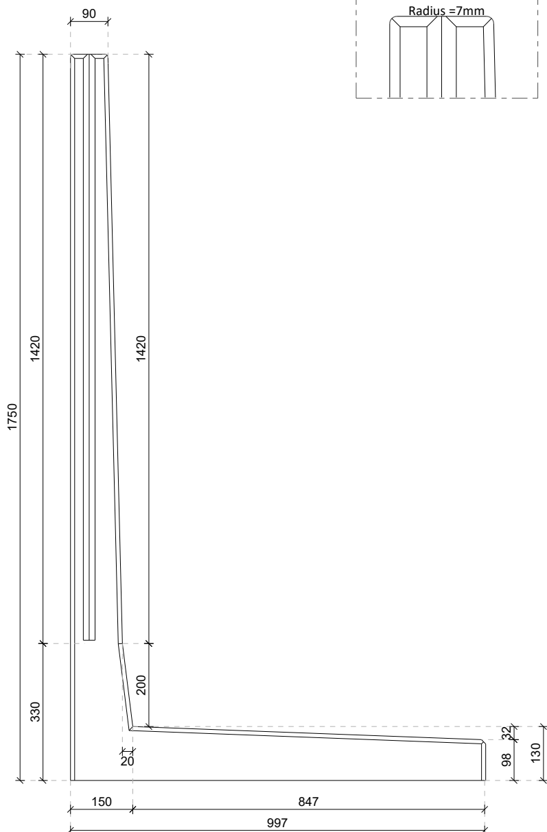
Afgeronde bovenzijde
